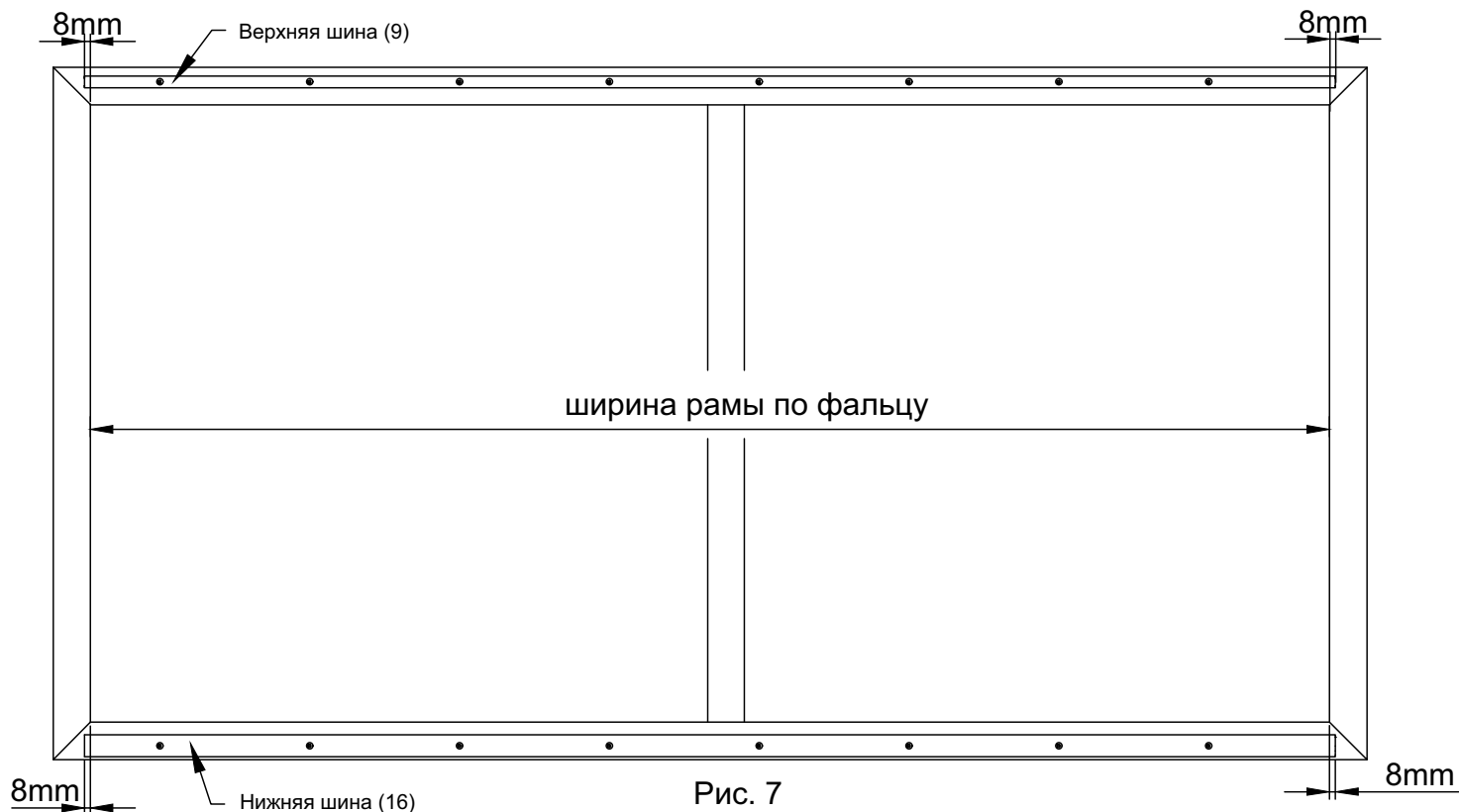
Шаблон Верхней шины (9)
